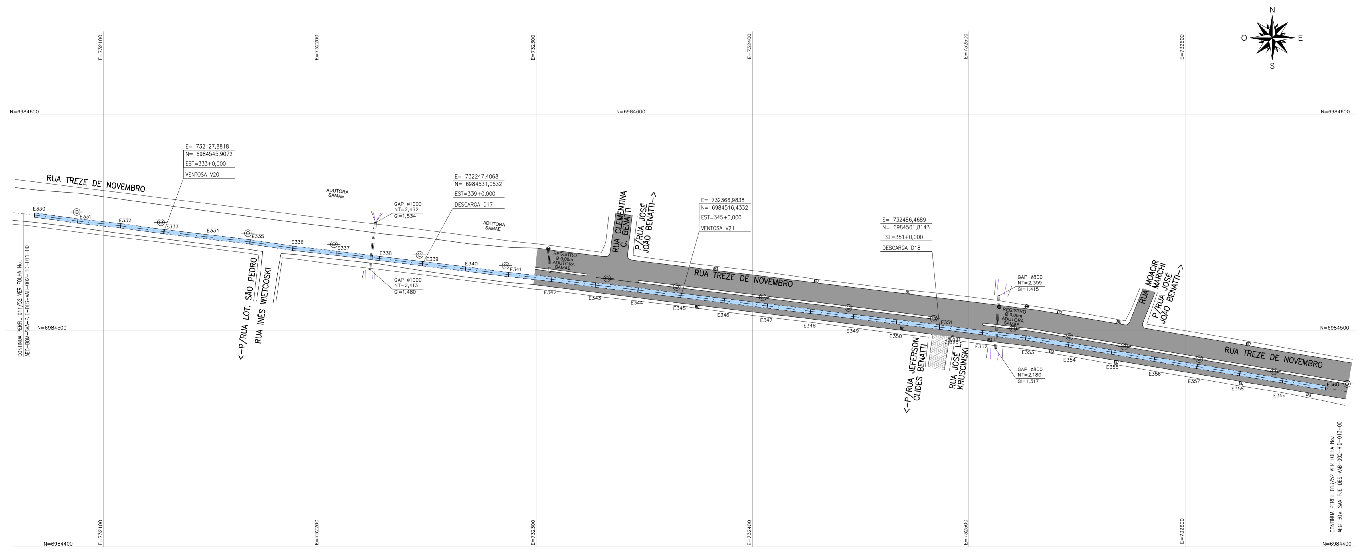
PLANTA 12/52 ADUTORA DE ÁGUA BRUTA ESCALA HORIZONTAL: 1:1000
