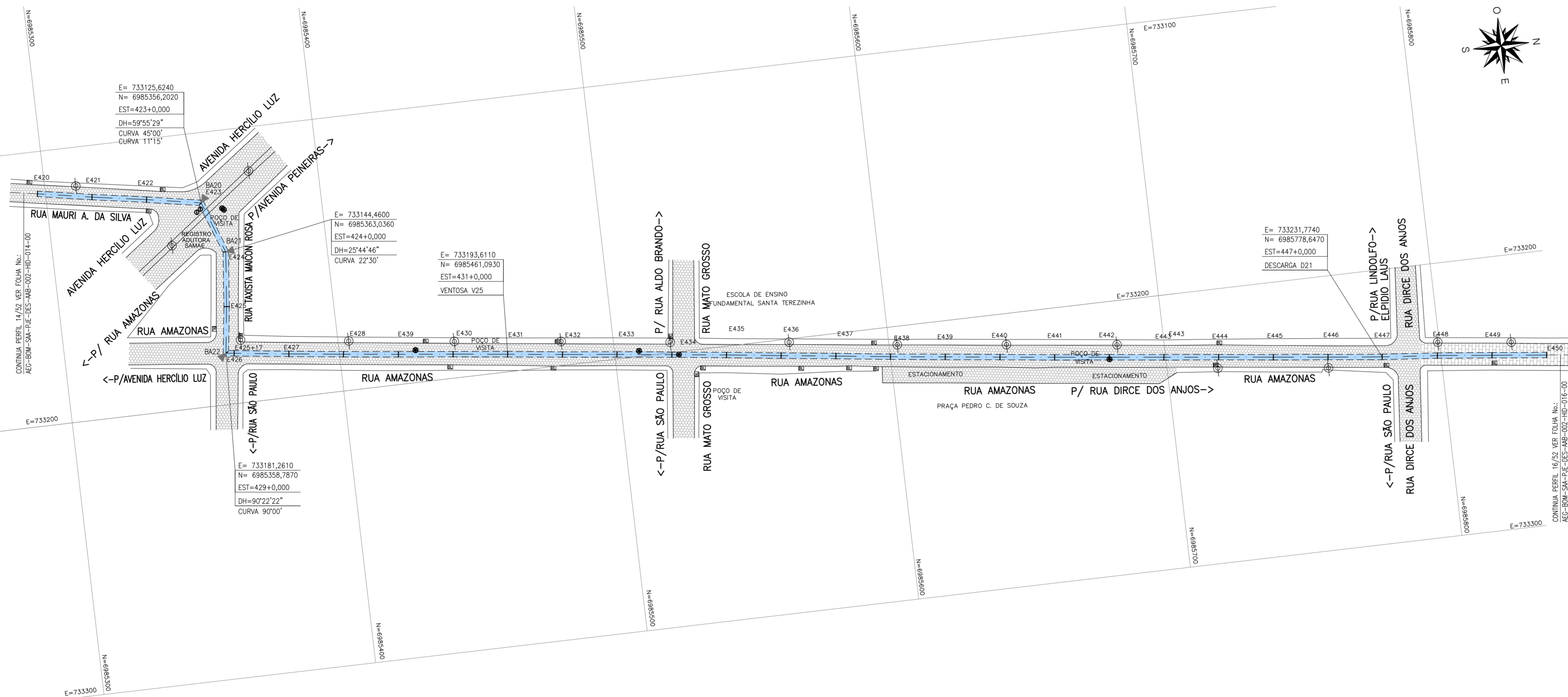
PLANTA 15/52 ADUTORA DE ÁGUA BRUTA ESCALA HORIZONTAL: 1:1000
