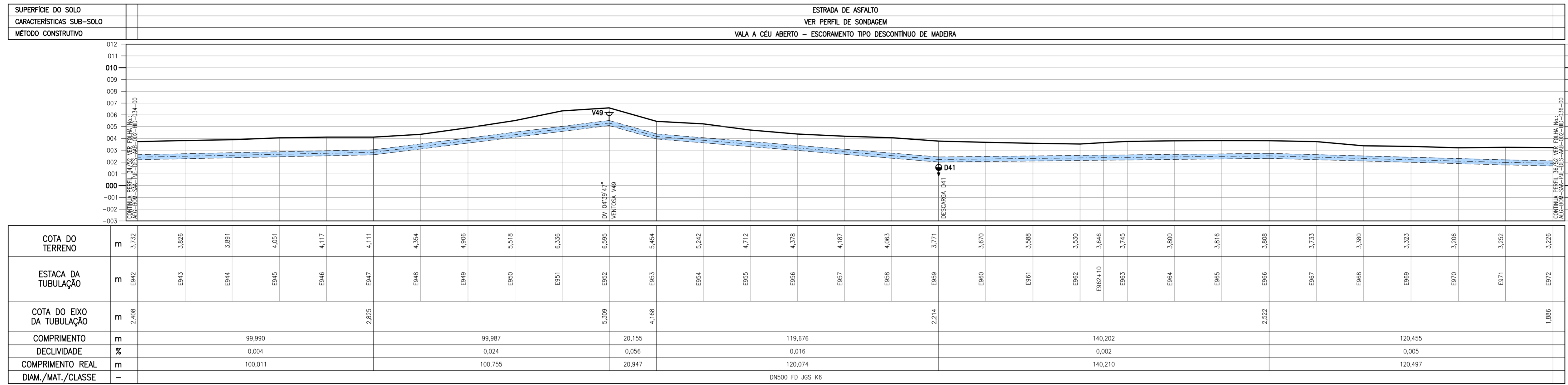
PERFIL 35/52 ADUTORA DE ÁGUA BRUTA ESCALA HORIZONTAL: 1:1000 ESCALA VERTICAL: 1:200
